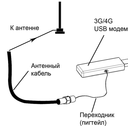
Схема 1 – Подключение антенны к USB модему
