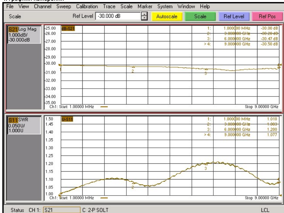
Графики для АЧХ - Log Mag, при отсчётном уровне равном -30 дБ, и для КСВ – SWR
